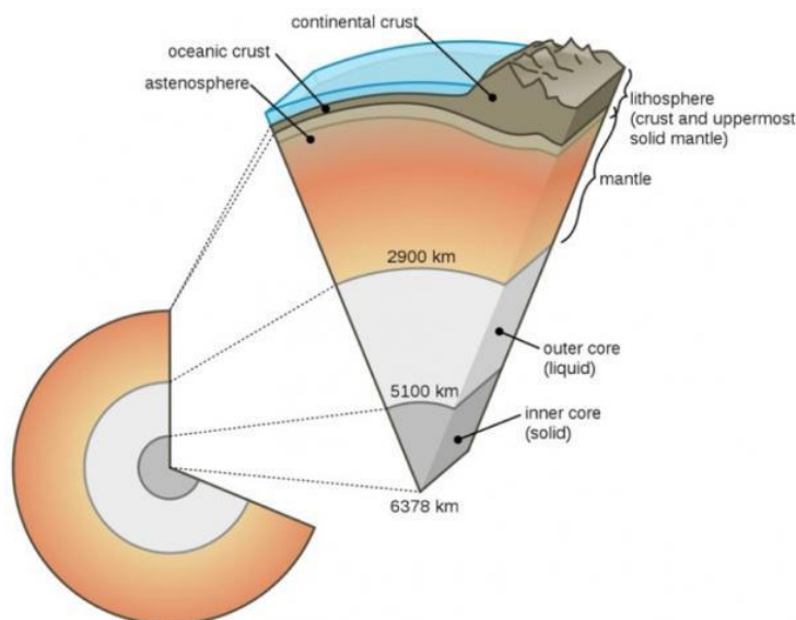
Diagram over den indre lagdeling af Jorden, der viser litosfæren over asthenosfæren (ikke i skala). (Nefronus / Public Domain )
